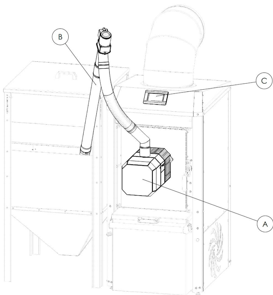
Ryc. 32. Lokalizacja części zamiennych w nagrzewnicy powietrza KIP.
