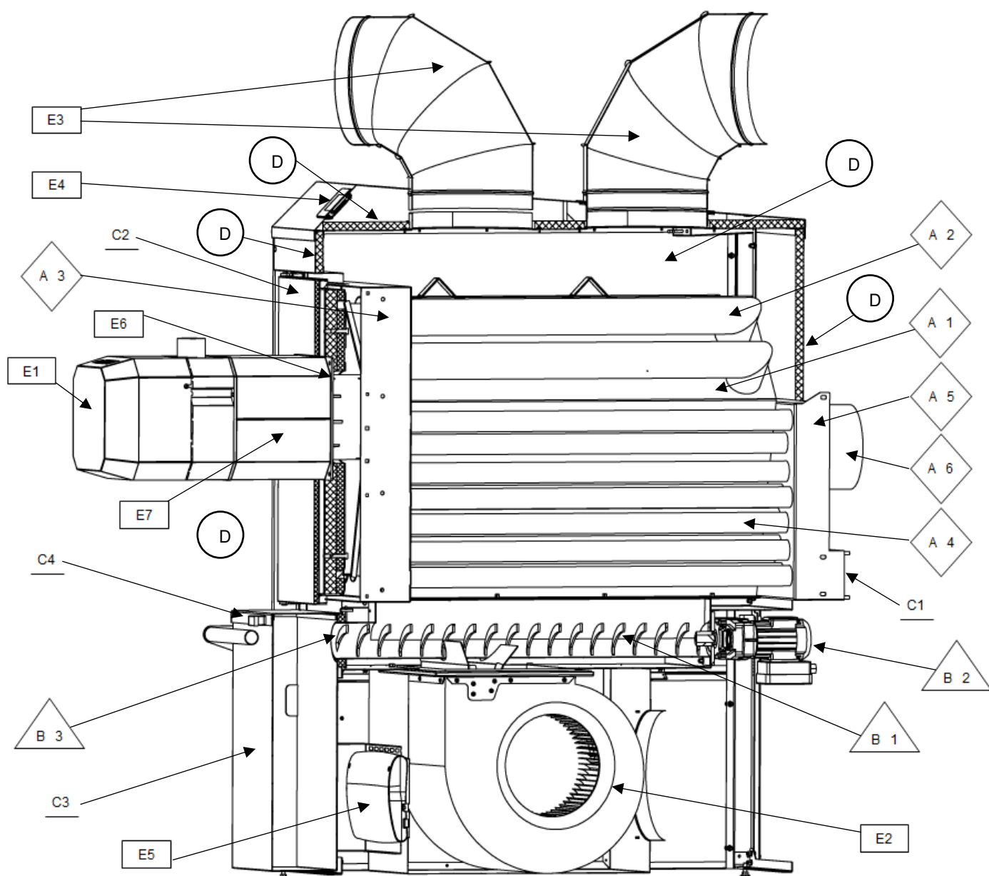
Ryc. 2. Budowa nagrzewnicy powietrza KIPi.
