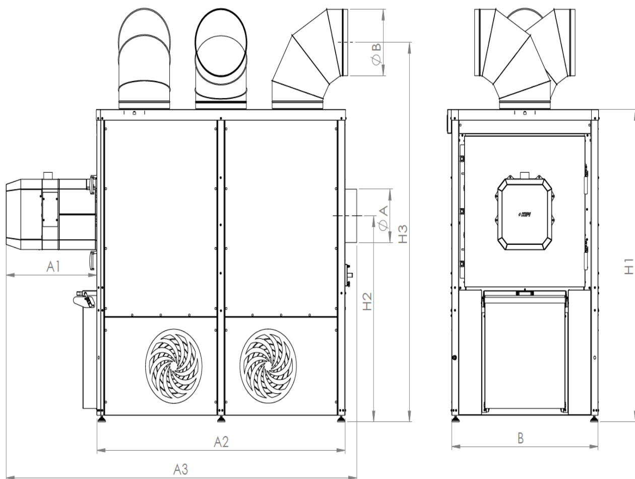
Ryc. 29. Wymiary gabarytowe nagrzewnicy powietrza KIPi, rysunek poglądowy urządzeń 250kW.
