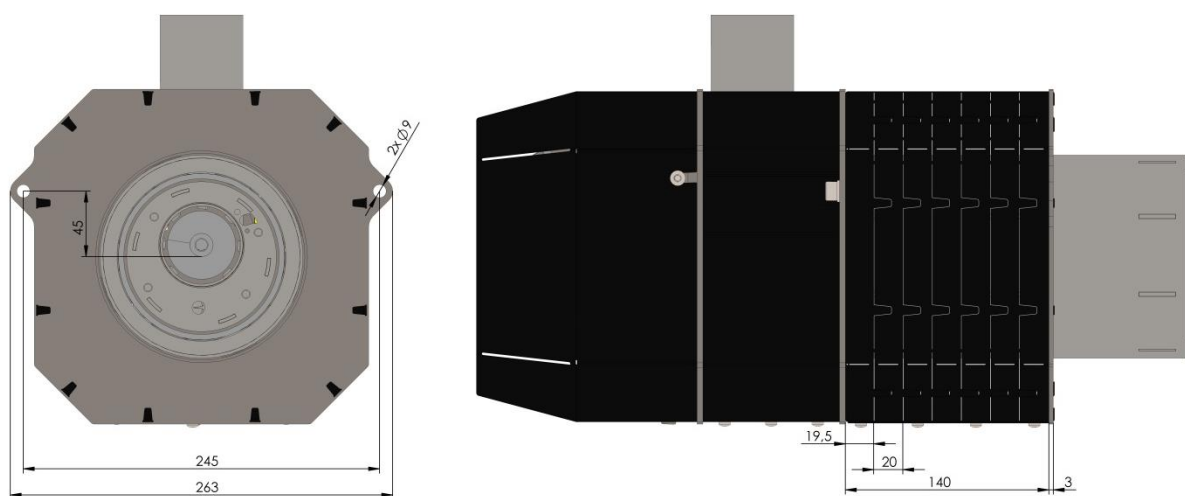
Rys. 24. Widok palnika 8-36 kW.
