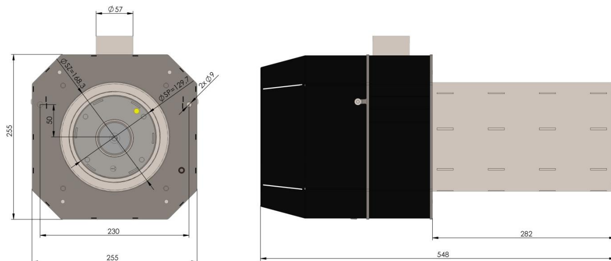
Rys. 26. Widok palnika 10-50kW.
