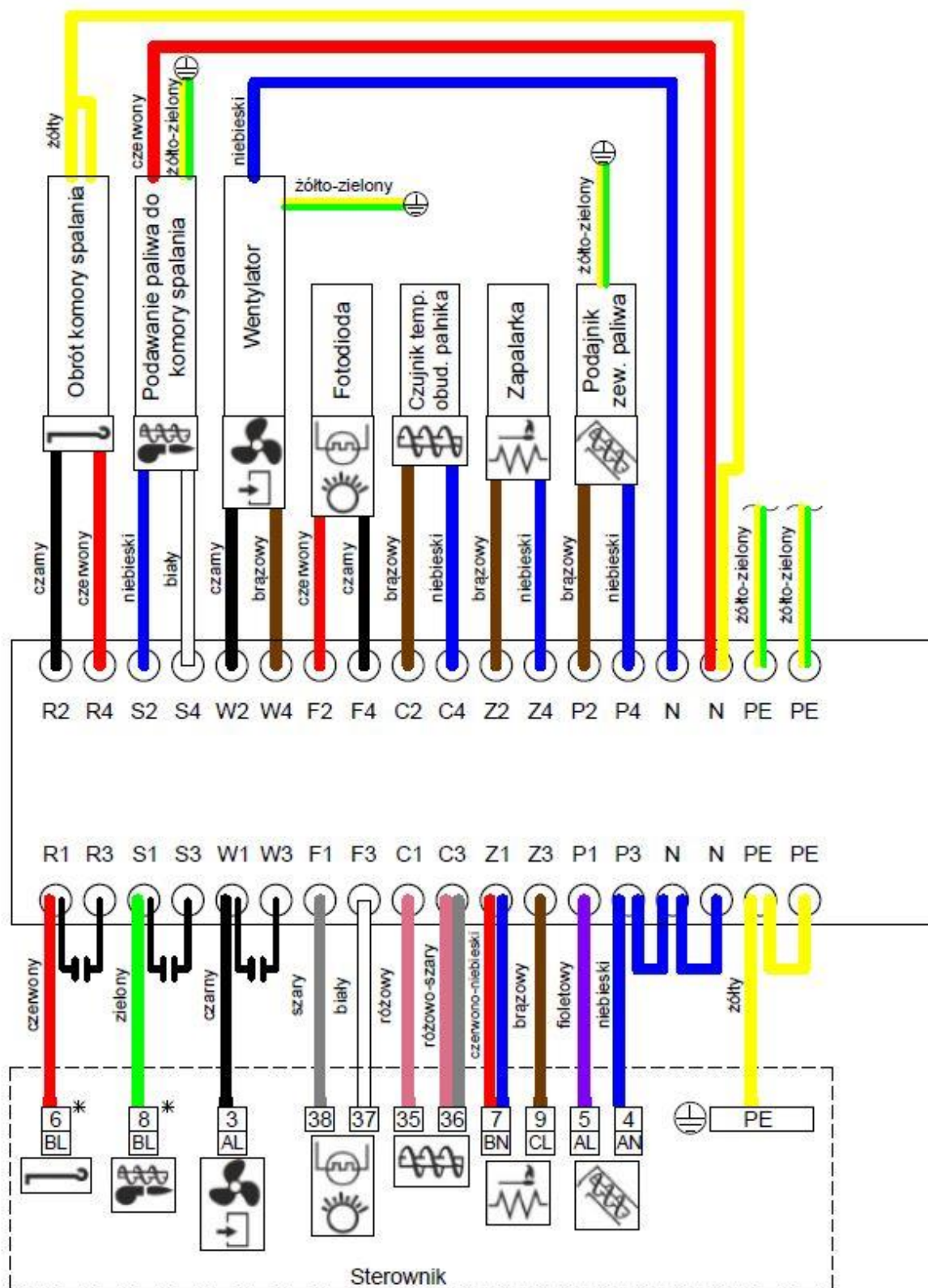
*Rys. 17. Schemat połączeń elektrycznych palnika z sterownikiem ecoMAX 850 w. 10.53. W przypadku połączenia z innym typem sterownika należy zweryfikować połączenia wg jego schematu elektrycznego.
