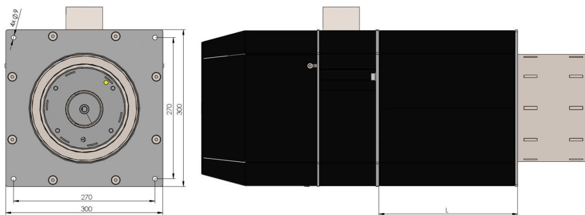
Rys. 19. Widok palnika 20-100 kW z płaszczem izolacyjnym i płytą montażową.
