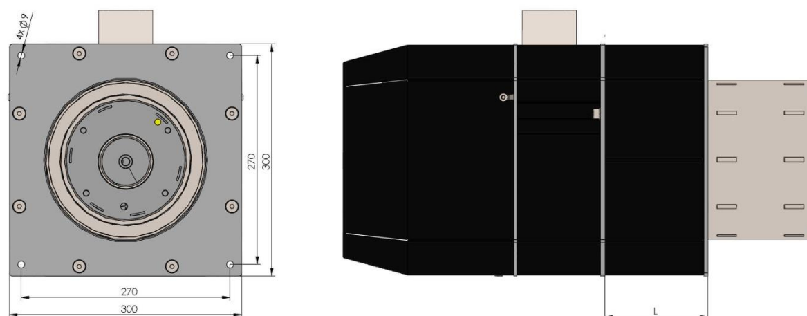
Rys. 16. Widok palnika 15-70 kW.
