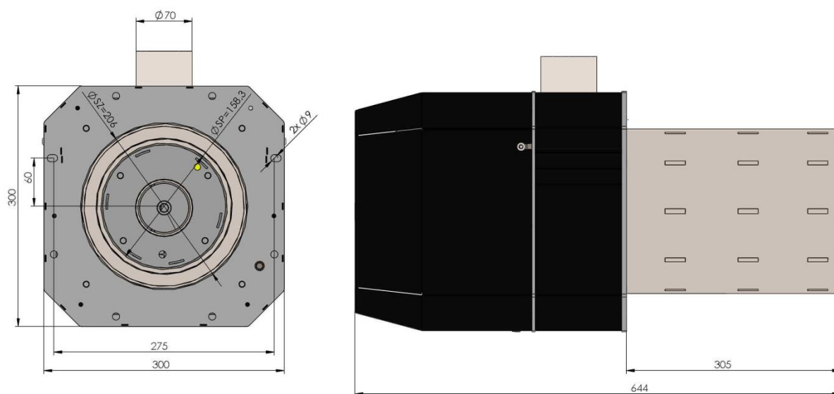
Rys. 16. Widok palnika 15-70 kW.
