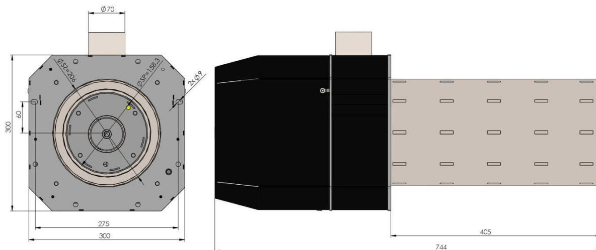
Rys. 18. Widok palnika 20-100 kW.
