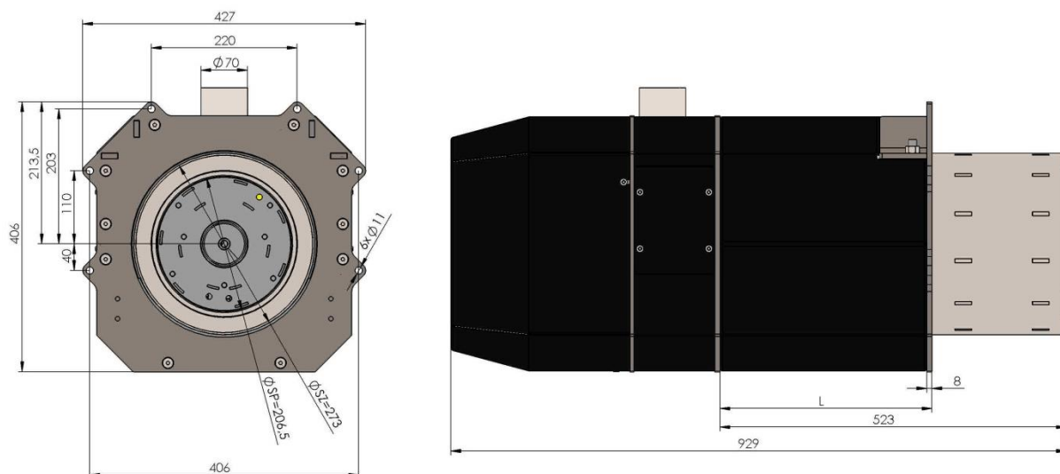
Rys. 19. Widok palnika 30-200 kW.
