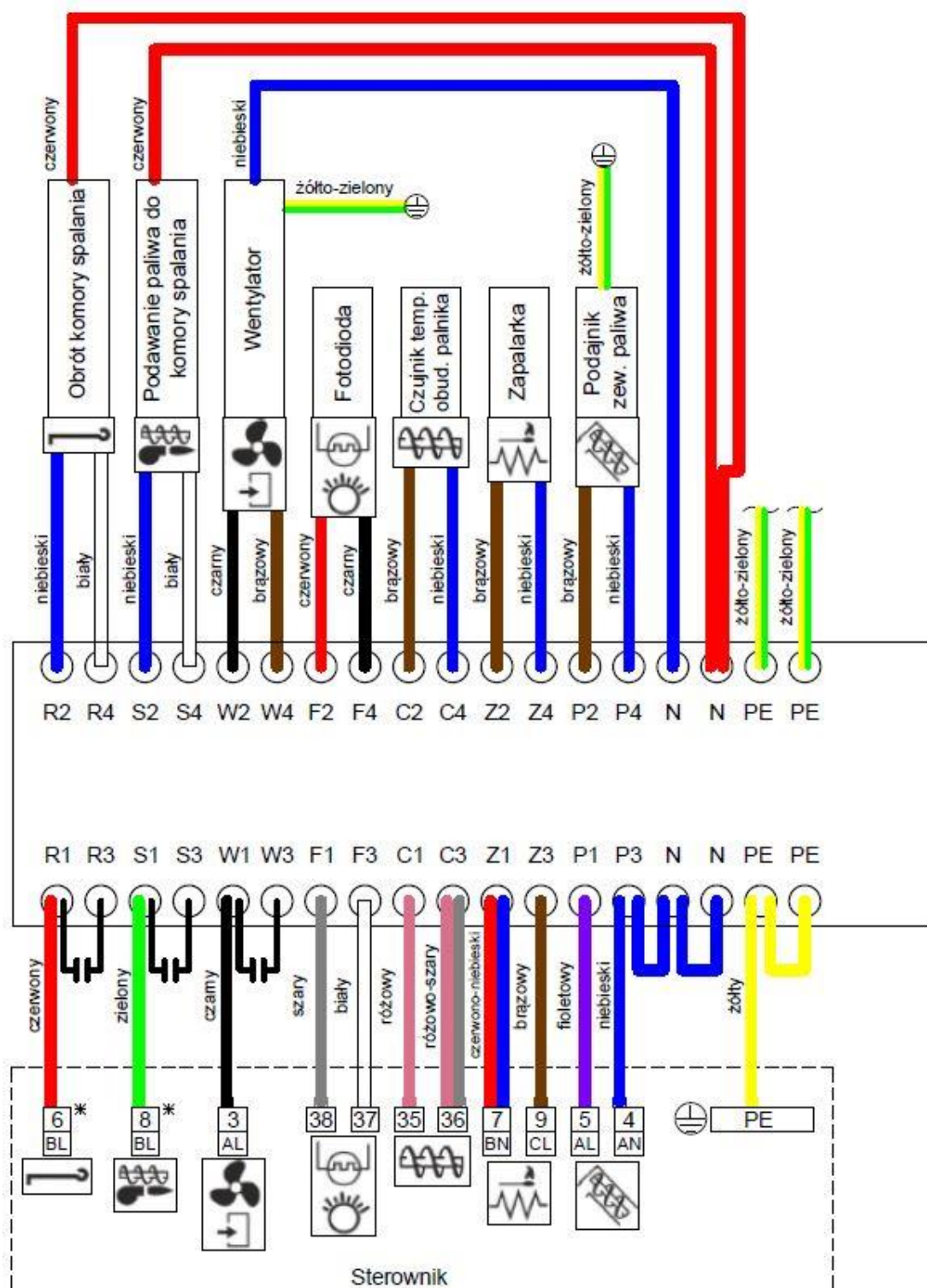
*Rys. 16. Schemat połączeń elektrycznych palnika z sterownikiem ecoMAX 850 w. 10.53. W przypadku połączenia z innym typem sterownika należy zweryfikować połączenia wg jego schematu elektrycznego.
