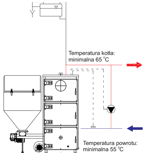
Termiczne zabezpieczenie temperatury powrotu kotła poprzez wykorzystanie pompy kotła
