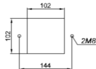
Wymiary otworu montażowego
