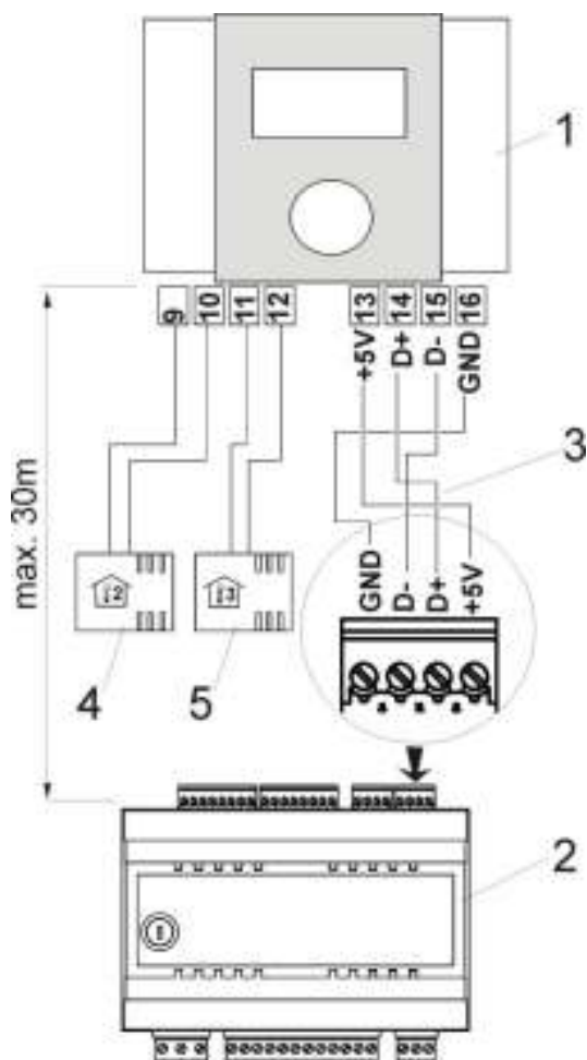
Rys. 8.3 Schemat podłączenia elektrycznego (czteroprzewodowego), gdzie: 1 – panel pokojowy ecoSTER200, 2 – regulator ecoMAXX800R2, ecoMAXX800T2, ecoMAX800P1, ecoMAX800P2, 3 – przewód łączący, 4 czujnik pokojowy termostatu 2 typ CT7, 5 – czujnik pokojowy termostatu 3 typ CT7.
