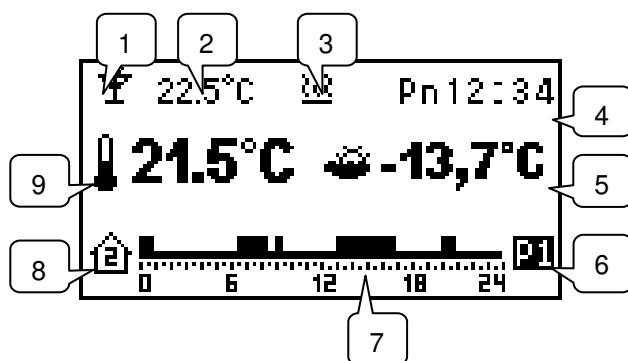
Rys. 7.1 Przykładowy widok ekranu głównego dla termostatu 2
