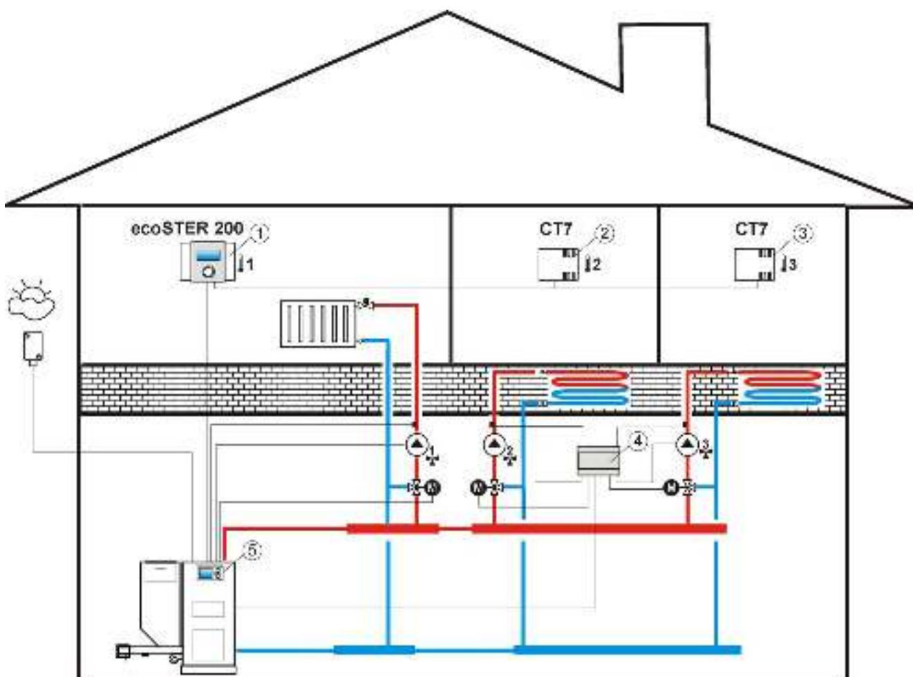
Rys. 8.9 2 Schemat współpracy ecoSTER z ecoMAX800, gdzie: 1 - ecoSTER200, 2- czujnik pokojowy termostatu 2 typ CT7, 3- czujnik pokojowy termostatu 3 typ CT7, 4- moduł MX.01 (rozszerza system o 2 obiegi grzewcze), 5 - regulator ecoMAX800R lub T.
