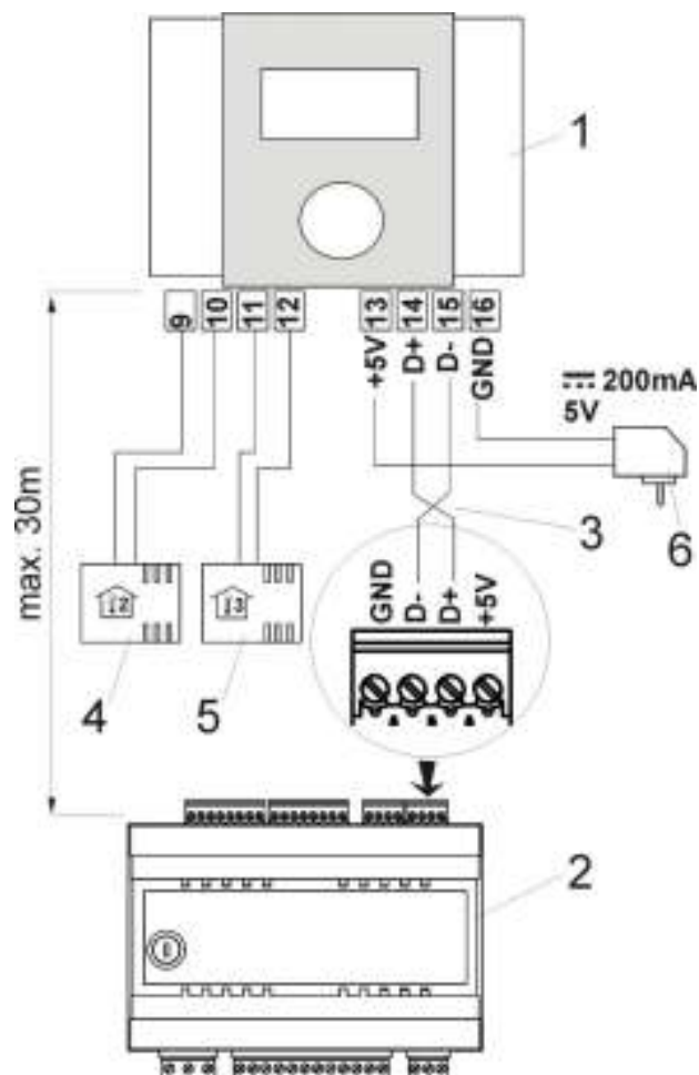
Rys. 8.4 Schemat podłączenia elektrycznego (dwuprzewodowe), gdzie: 1 – panel pokojowy ecoSTER200, 2 – regulator ecoMAXX800R2, ecoMAXX800T2, ecoMAX800P1, ecoMAX800P2, 3 – przewód łączący, 4 czujnik pokojowy termostatu 2 typ CT7, 5 – czujnik pokojowy termostatu 3 typ CT7, 6 – zasilacz 5V.
