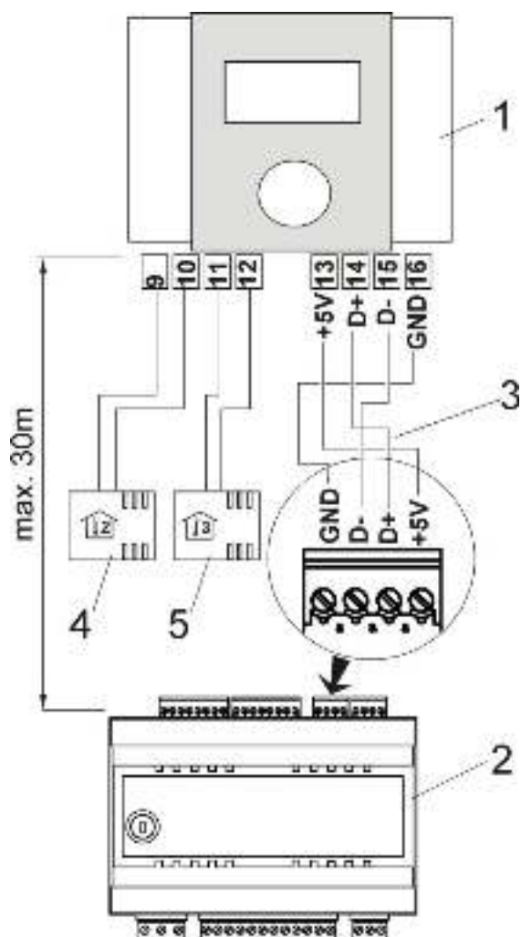
Rys. 8.5 Schemat podłączenia elektrycznego, gdzie: 1 – panel pokojowy ecoSTER200, 2 – regulator ecoMAX800R1 lub ecoMAX800T1, 3 – przewód łączący, 4 czujnik pokojowy termostatu 2 typ CT7, 5 – czujnik pokojowy termostatu 3 typ CT7.
