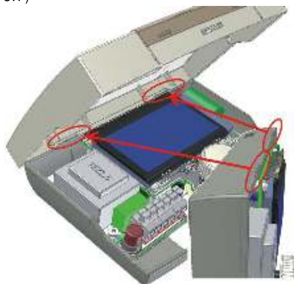
Rys. 8.7 Zamknięcie obudowy krok pierwszy, (rysunek poglądowy)
